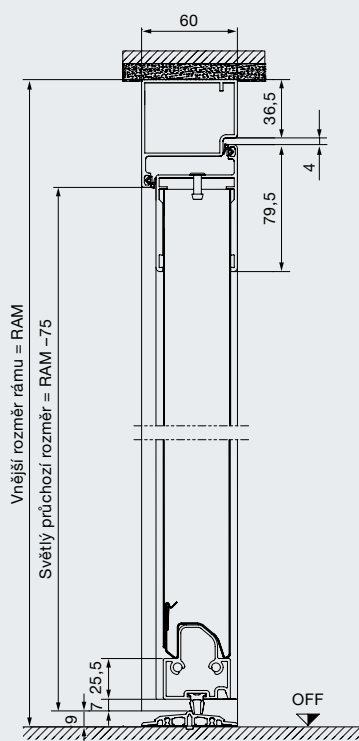
Svislý řez NT60-2
